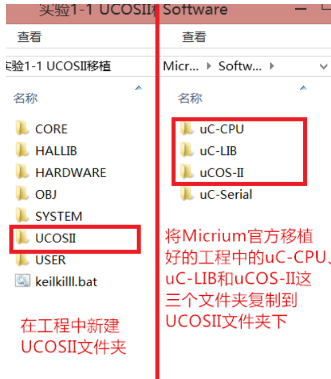
图 1.2.1.1 新建 UCOSII 文件夹并添加相应文件
