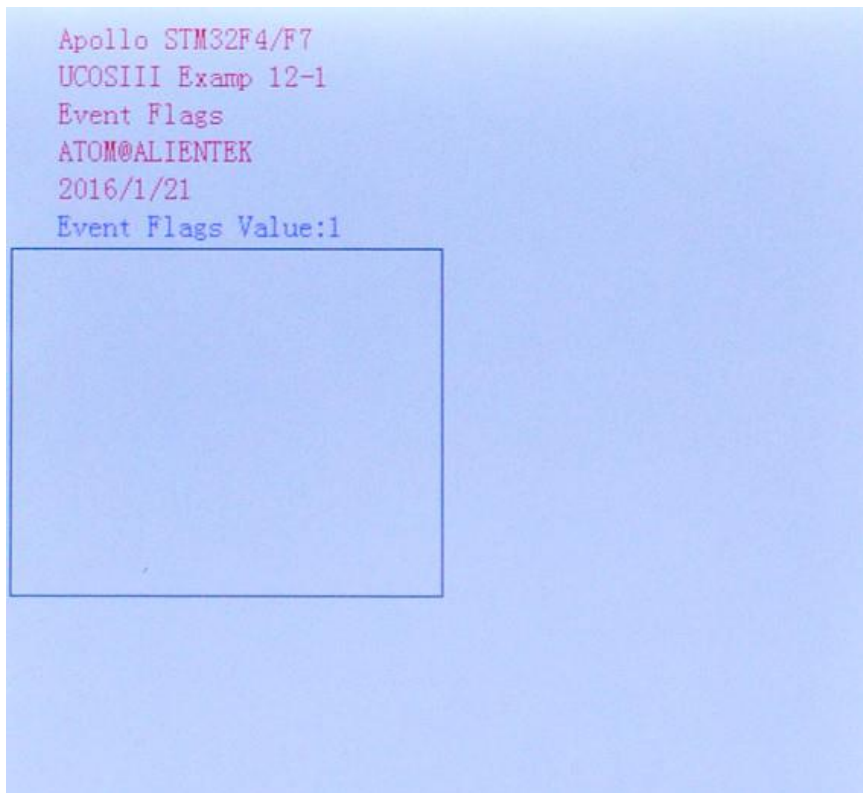
图 12.3.2 按下 KEY0 后的 LCD 界面
