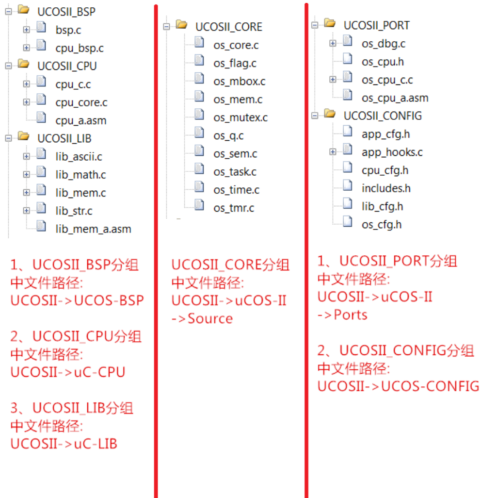
图 1.2.1.5 添加完成后的工程
