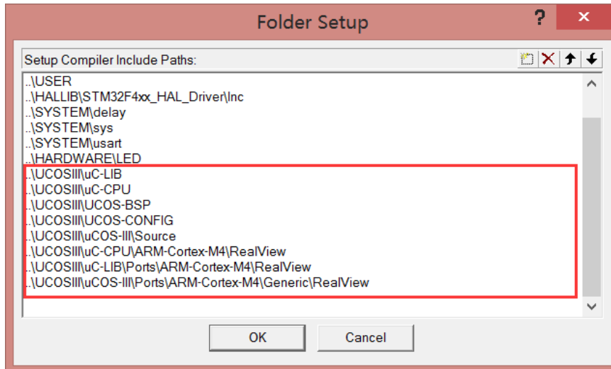
图 4.3.1.7 添加相应头文件
