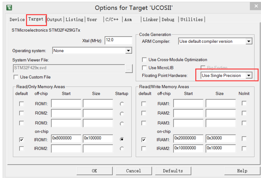
图 1.2.6.2 选择使用 FPU(单精度)
