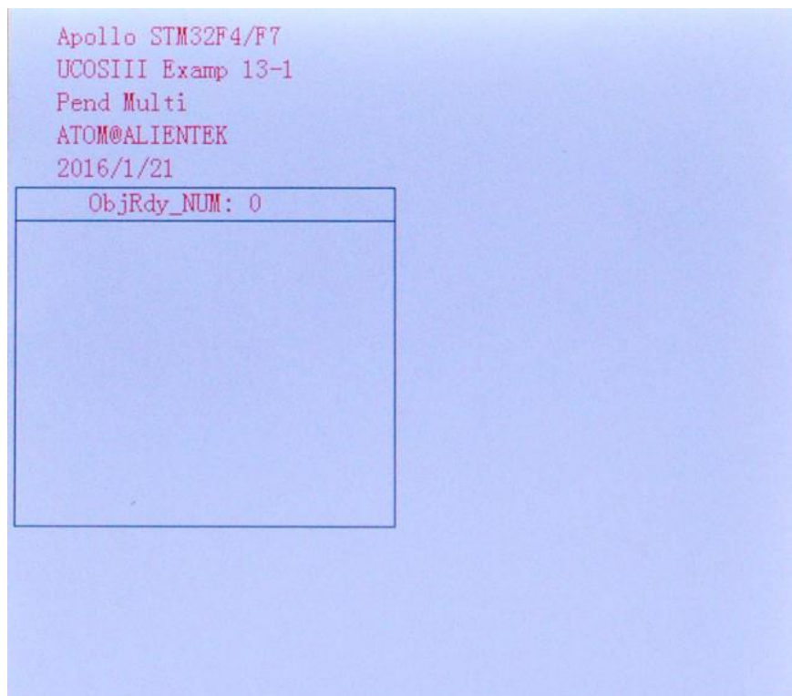
图 13.3.1 LCD 显示图
