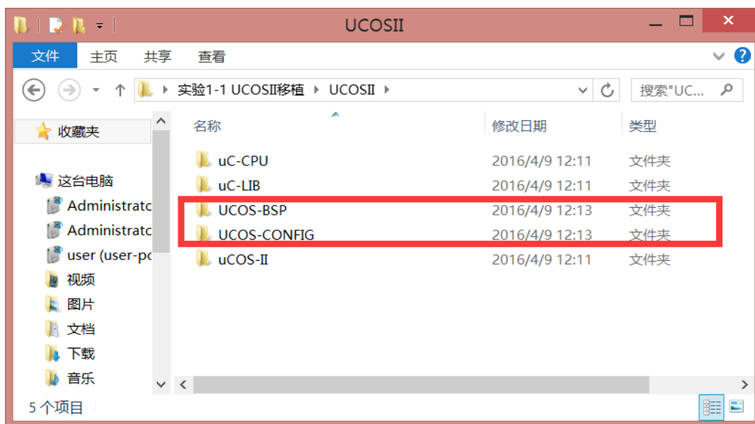
图 1.2.1.2 创建文件夹
