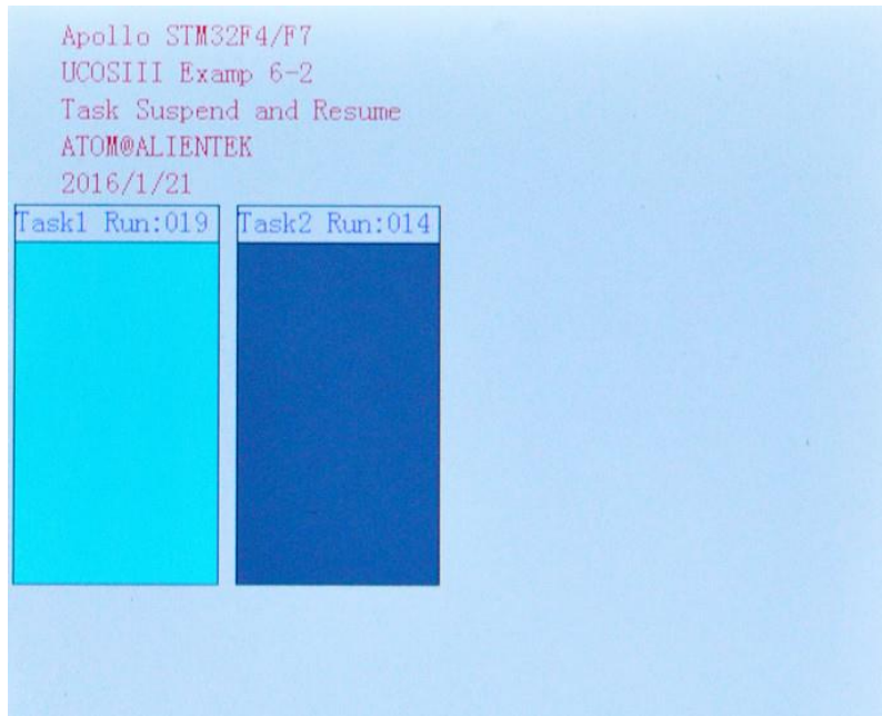
图 6.2.2 任务 2 恢复
