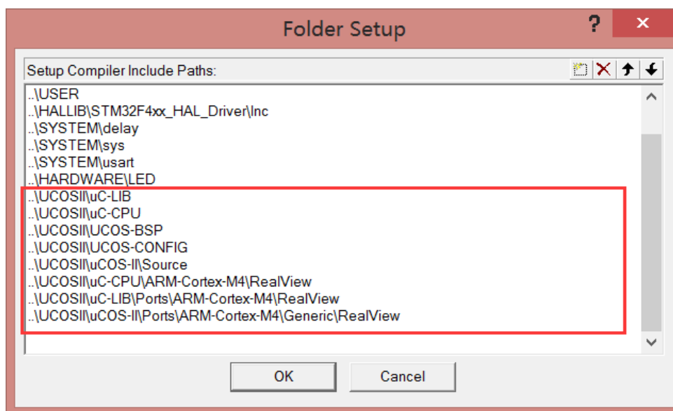
图 1.2.1.5 添加完成后的工程
