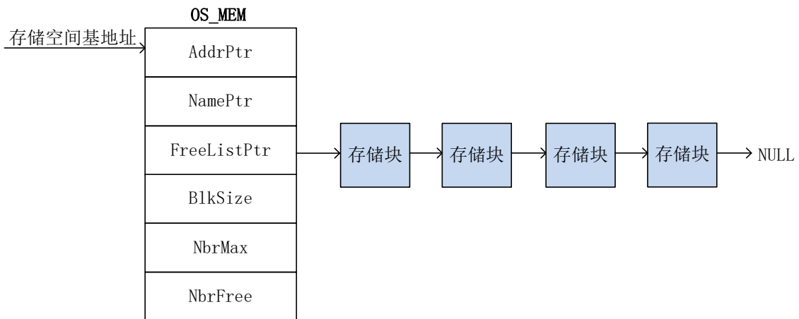
图 14.2.1 创建好的存储分区
