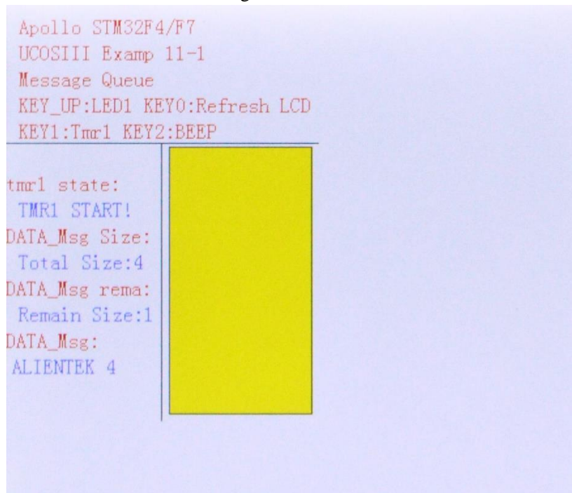
图 11.3.3 开启定时器 1
