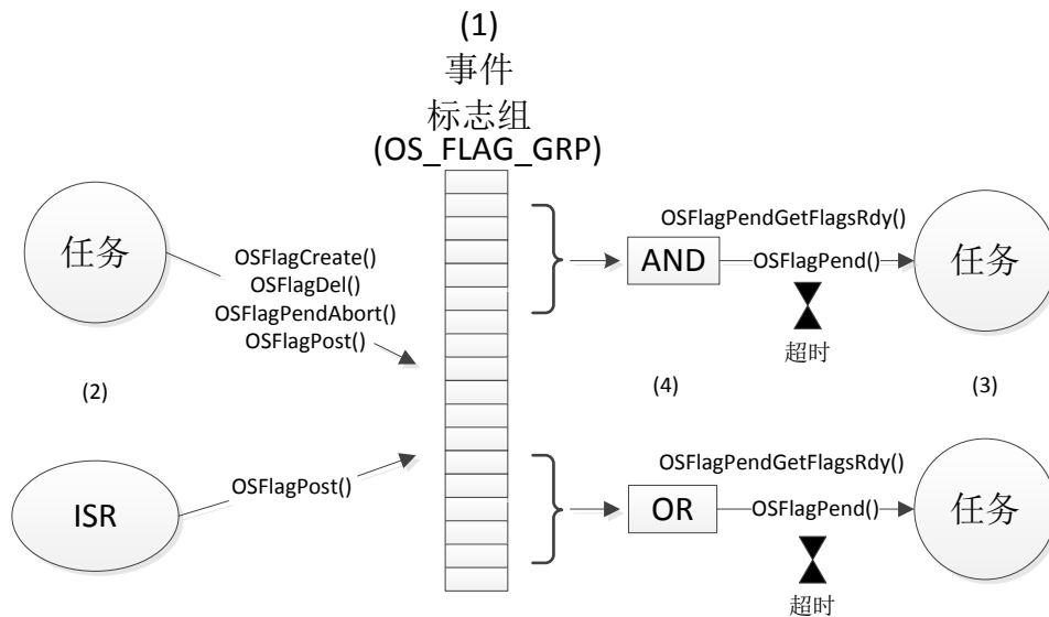
图 12.1.1 事件标志组
