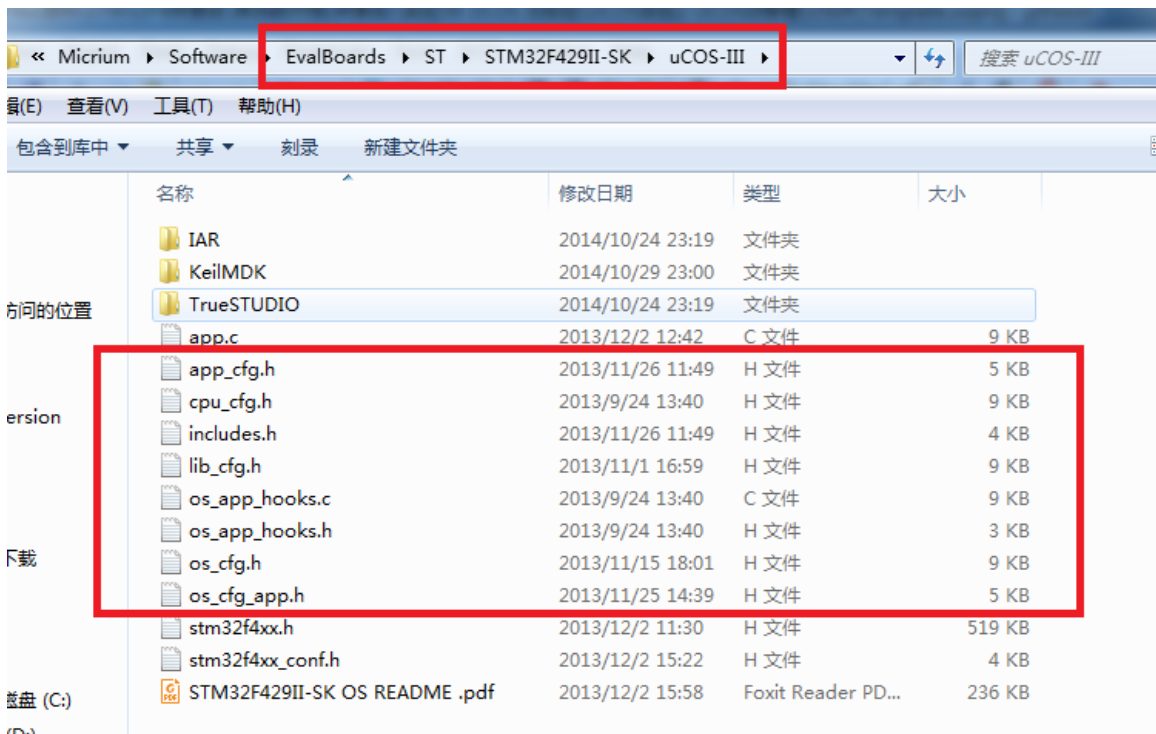
图 4.2.5 EvalBoards 文件
