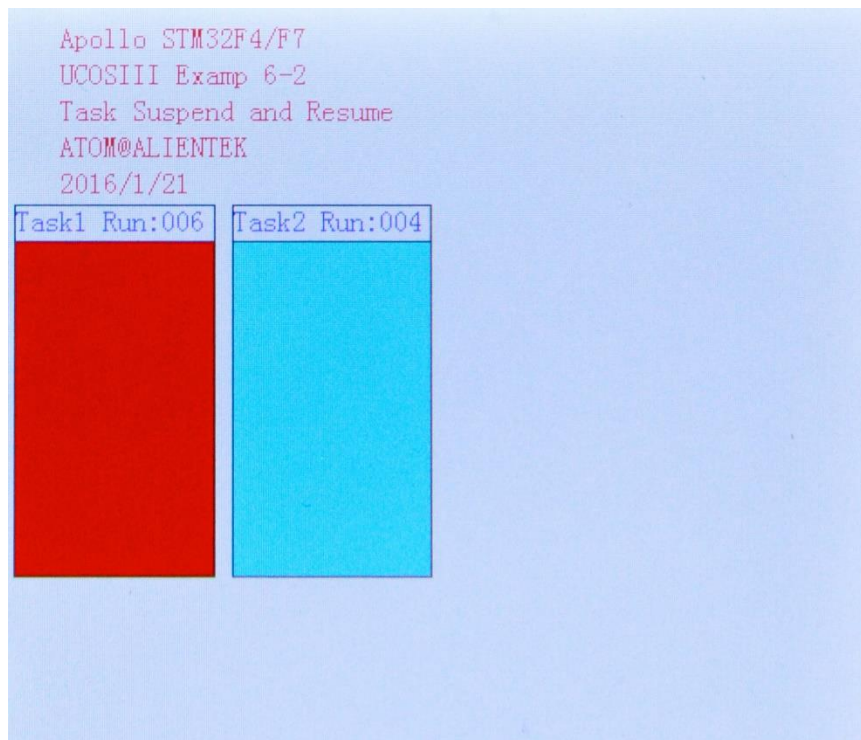
图 6.2.1 任务 2 被挂起
