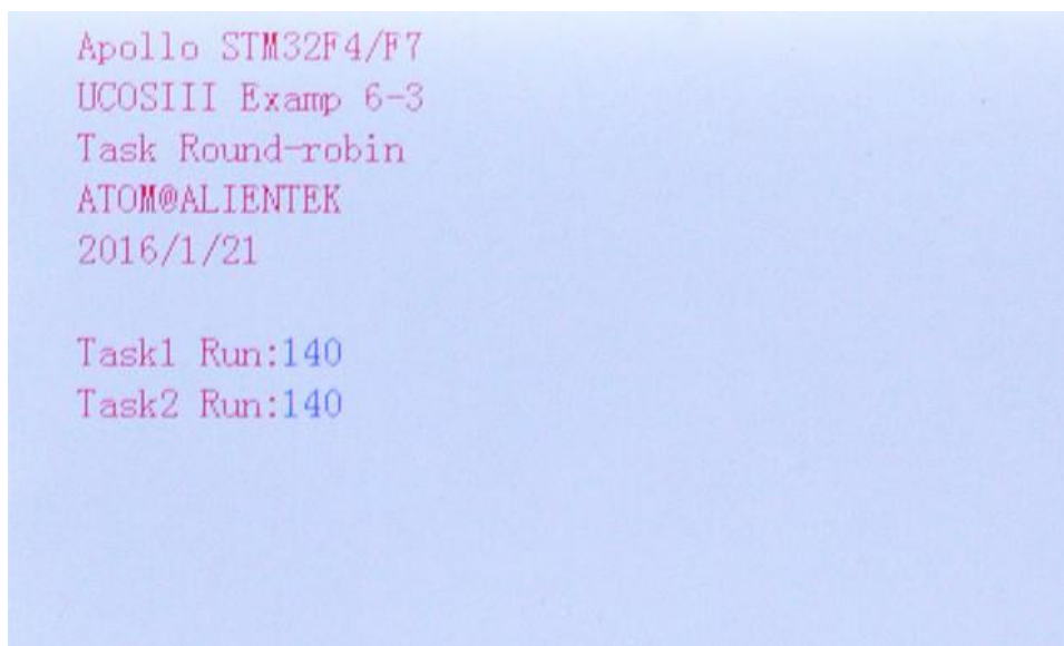
图 6.3.1 LCD 显示
