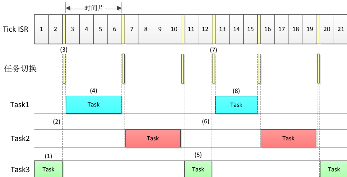
图 5.6.1 轮转调度
