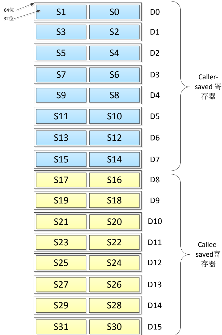
图 2.3.1 浮点寄存块
