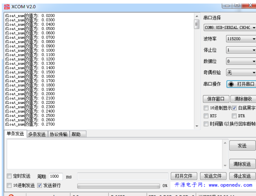
图 1.4.1 串口输出
